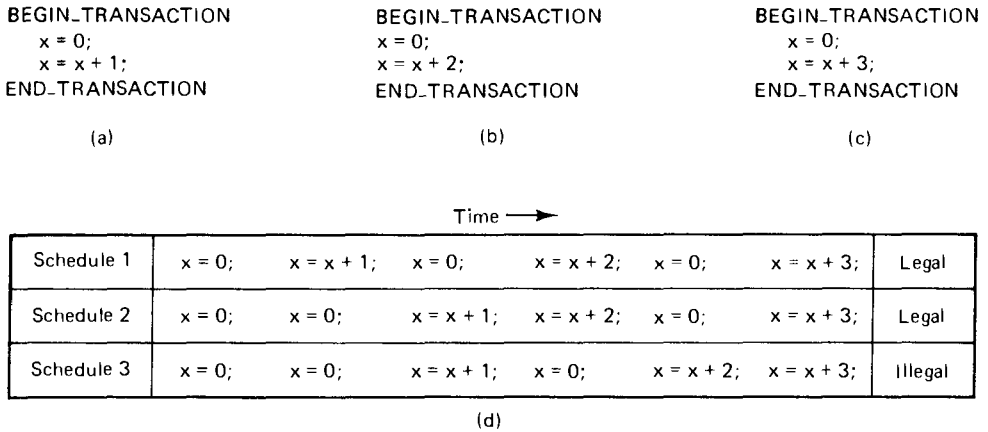
Fig. 3-17. (a)-(c) Three transactions. (d) Possible schedules.
