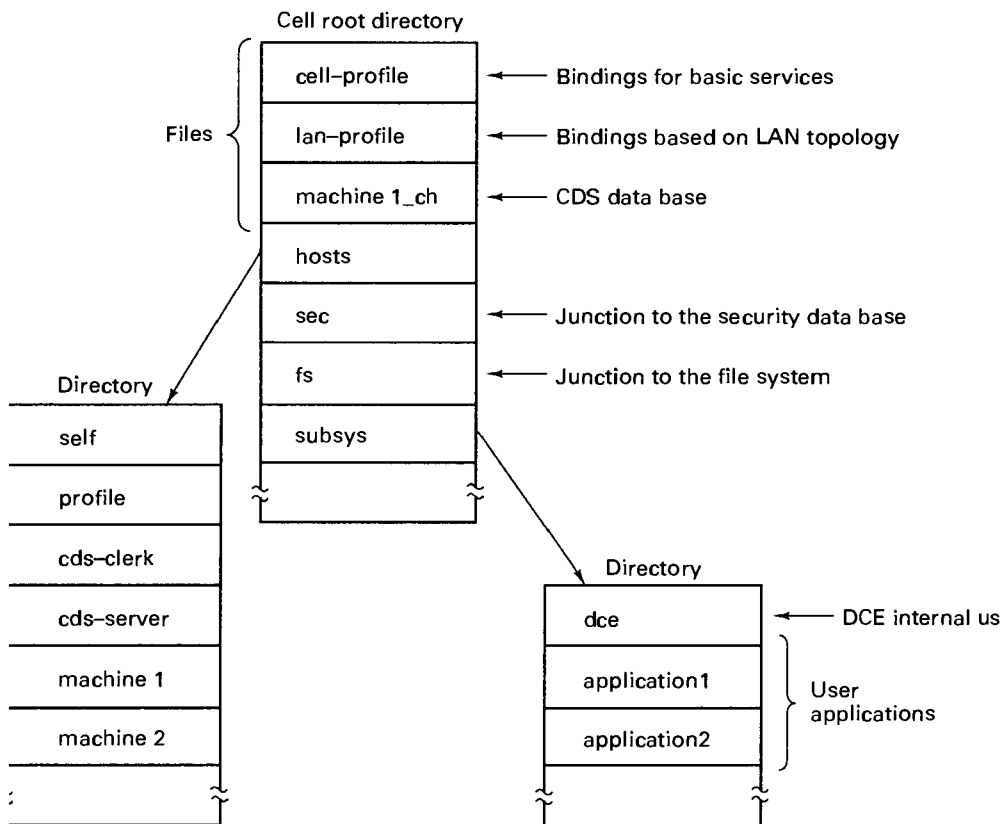
Fig. 10-20. The namespace of a simple DCE cell.
